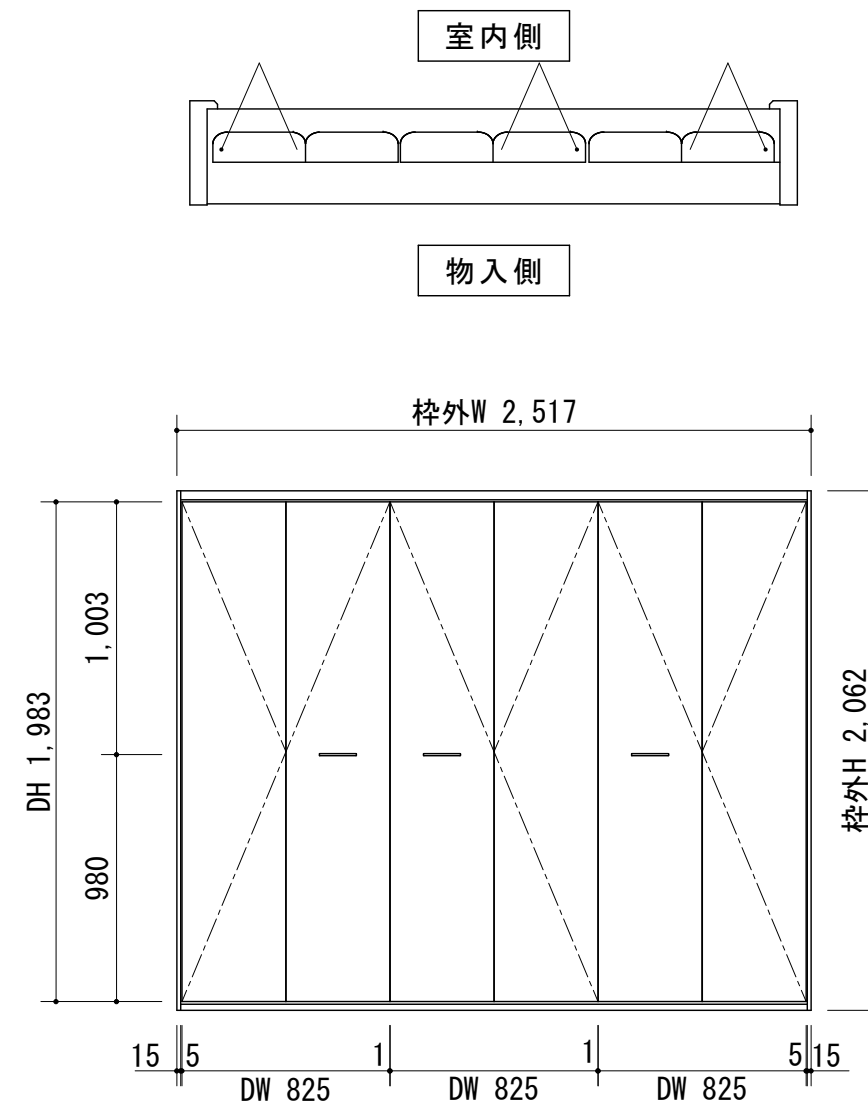
正面図
